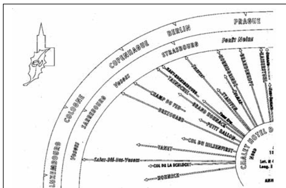
Partie du dessin ayant servi à l'étude et à la fabrication de la table d'orientation par le fondeur.
